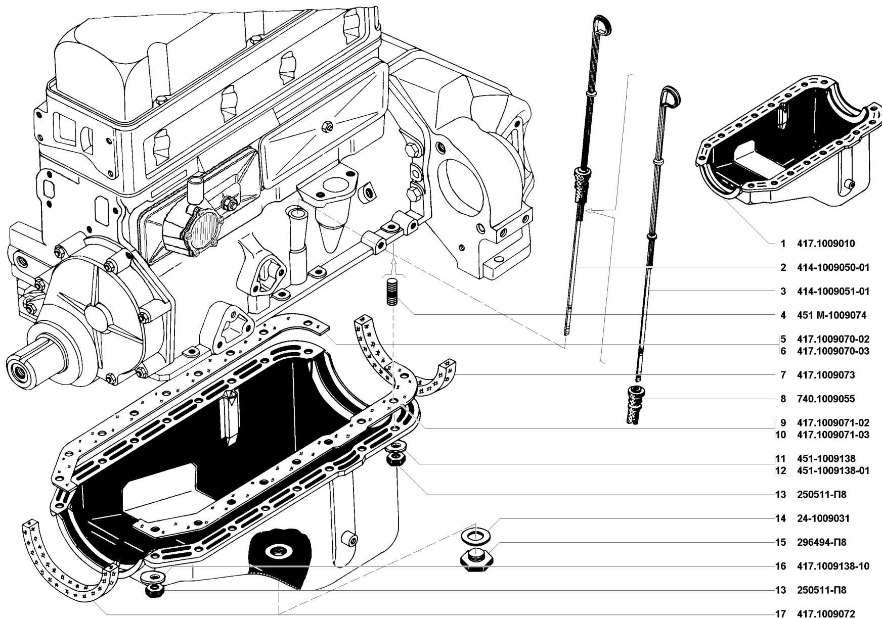
Рис. 11. Картер масляный (1009)
